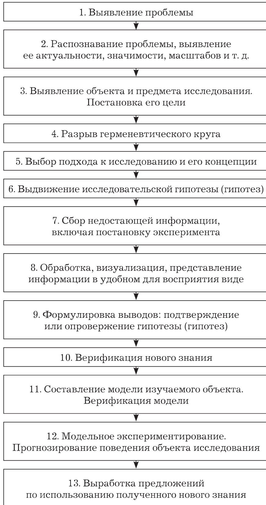
Рис. 1. Обобщенная схема исследования
