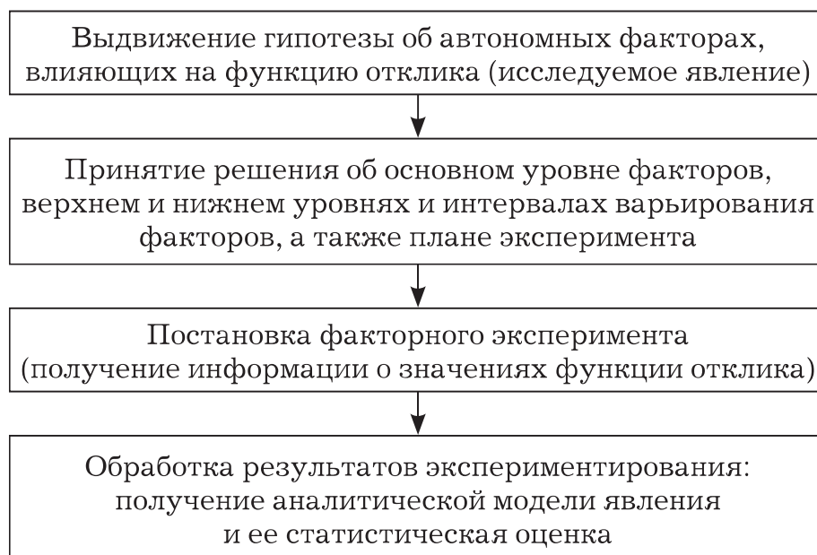
Рис. 34. Примерный алгоритм планирования эксперимента
