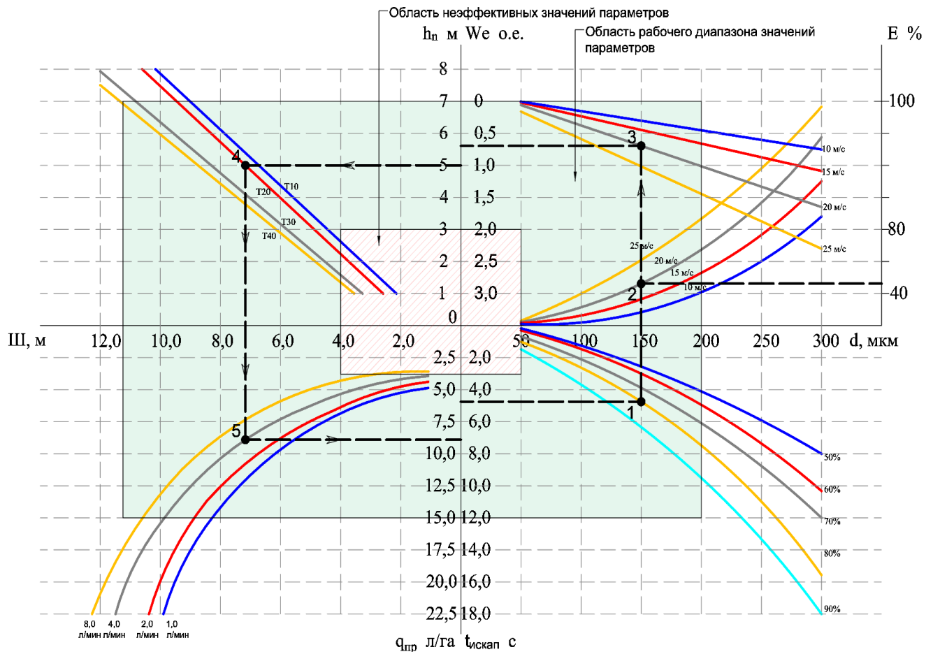
Рисунок 2.23 – Номограмма расчета параметров опрыскивания с БПЛА
