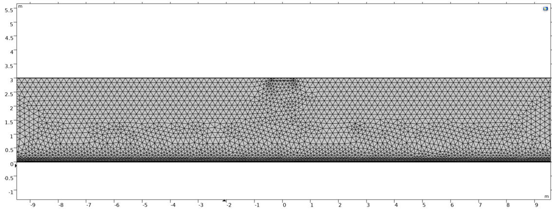
Рисунок 2.24 – Сетка моделирования
