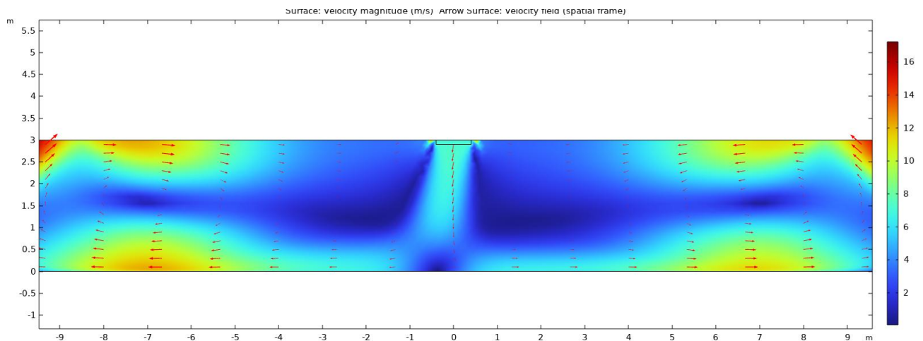
Рисунок 2.25 – Изображение результатов моделирования распространения воздушных потоков на высоте 3 метра
