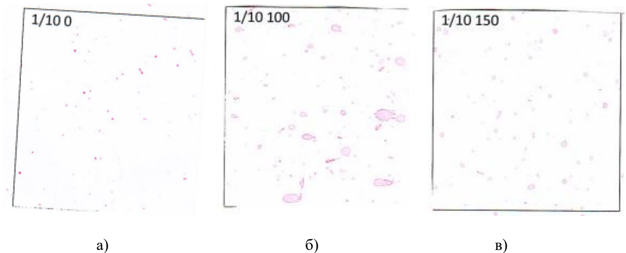
Рисунок 2.18 – Изображение учетных площадок для контроля качества опрыскивания на высоте полета 1 м при норме расхода 10 л/га
