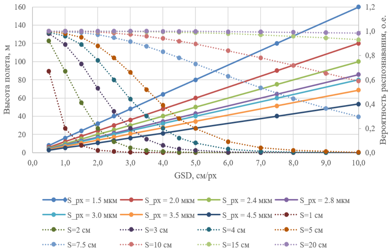
Рисунок 2.30 – Номограмма определения параметров аэрофотосъемки при различных значениях пикселя и размера объекта
