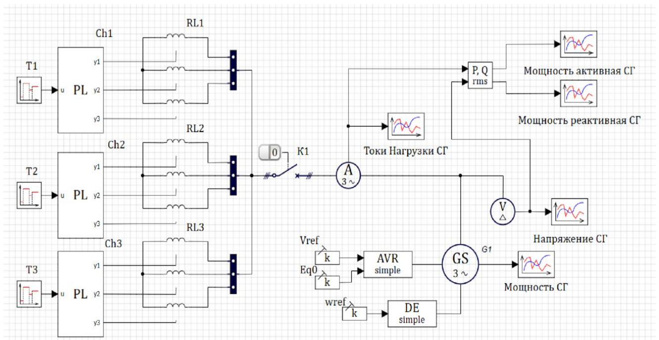
Рисунок 2.32 – Имитационная компьютерная модель автономного источника для БАС (модель выполнена в программе SimInTech)
