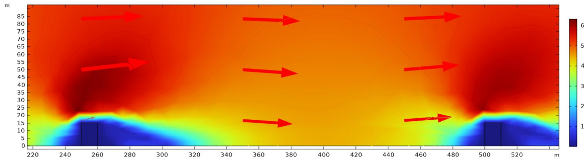
Рисунок 2.15 – Изображение результата моделирования распространения ветра между лесополосами при скорости 5 м/с
