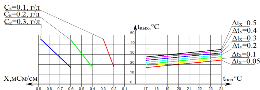
Рисунок 3.28 – Номограмма зависимости электропроводности от начальной температуры и температуры электролита на выходе из камеры при различных коэффициентах смещения температуры и конечной минерализации
