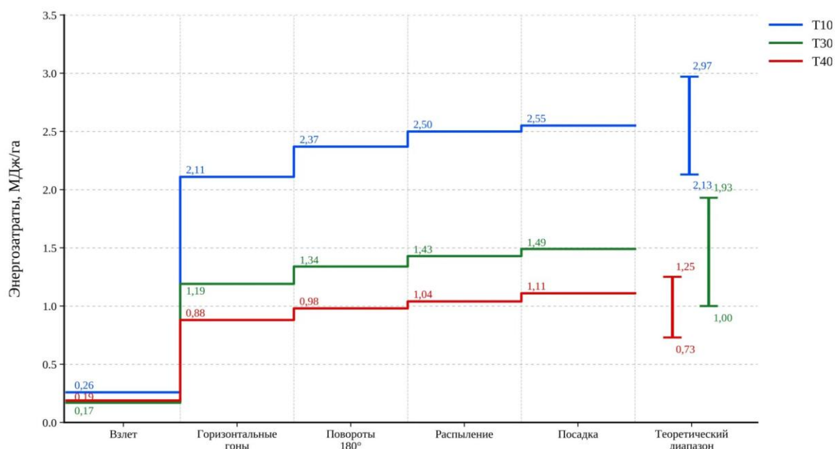
Рисунок 4.25 – Циклограмма нагрузок по БАС
