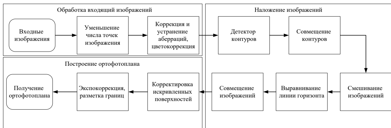
Рисунок 3.1 – Блок-схема алгоритма для обработки изображений и построения ортофотоплана
