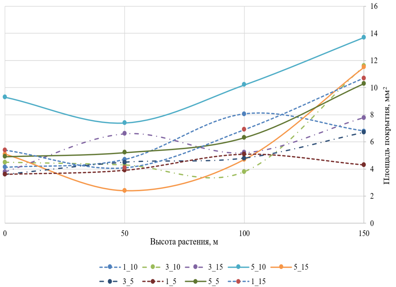
Рисунок 2.22 – Распределение площади покрытия капель по высоте растения
