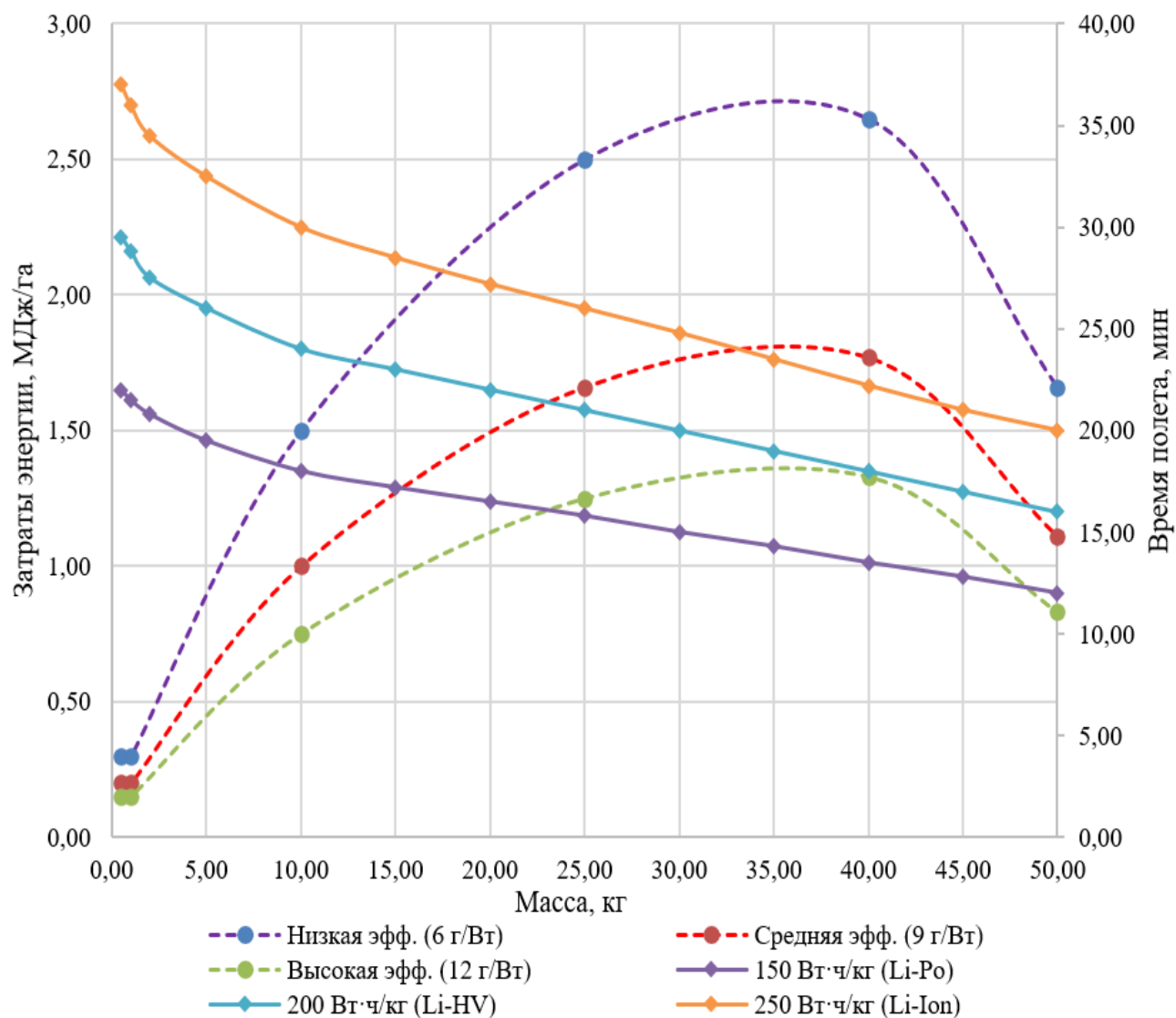
Рисунок 2.31 – График зависимости затрат энергии при различных типах винтов и времени при различных типах АКБ от массы БПЛА
