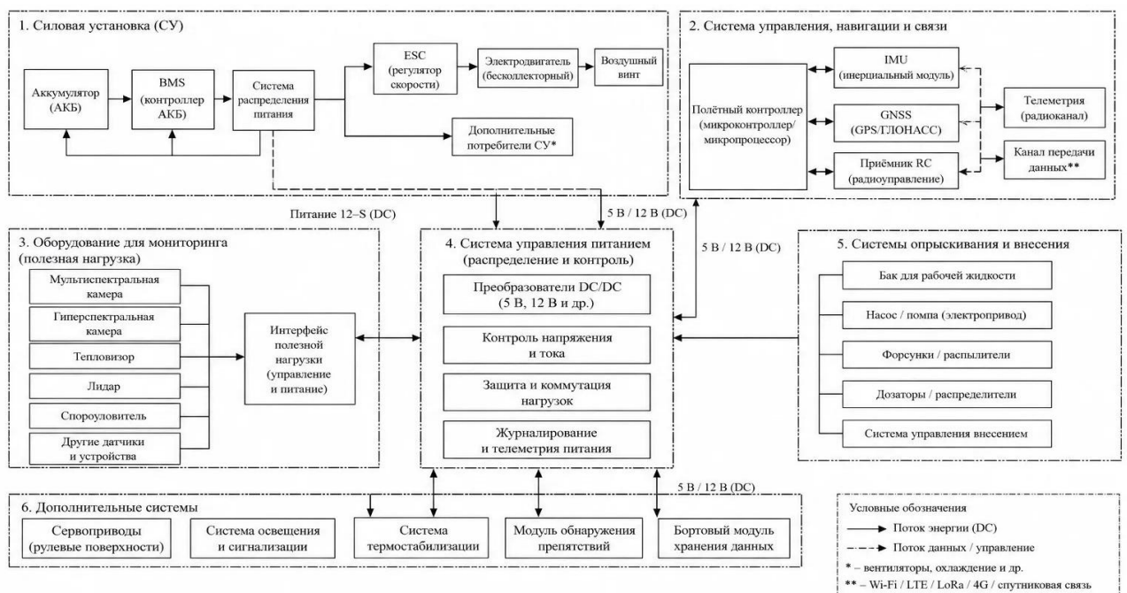
Рисунок 1.23 – Структурная энергетическая схема бортового оборудования БАС мультироторного типа
