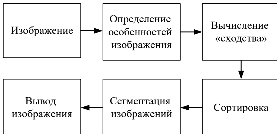
Рисунок 3.11 – Блок-схема алгоритма программы по сегментации областей изображений
