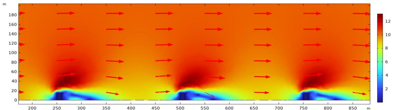
Рисунок 2.14 – Изображение результата моделирования распространения ветра между лесополосами при скорости 10 м/с
