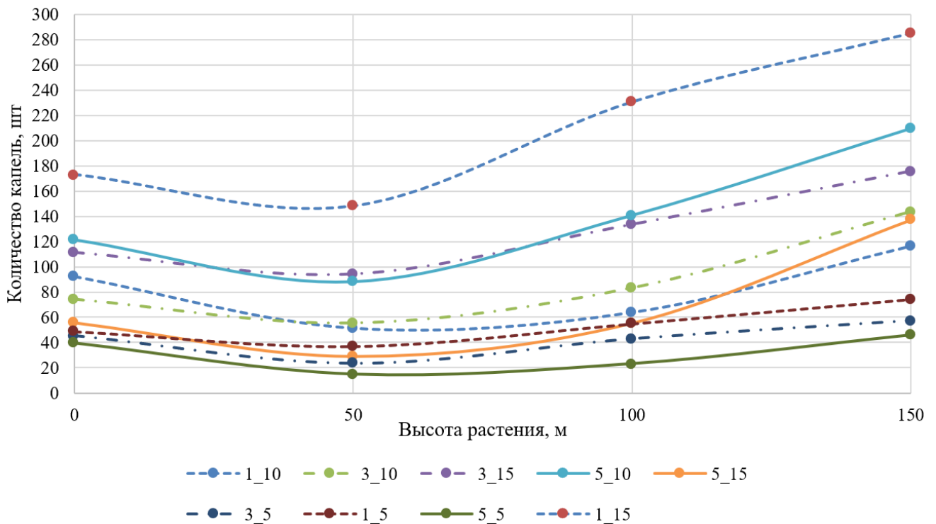
Рисунок 2.20 – График распределения капель по высоте растения
