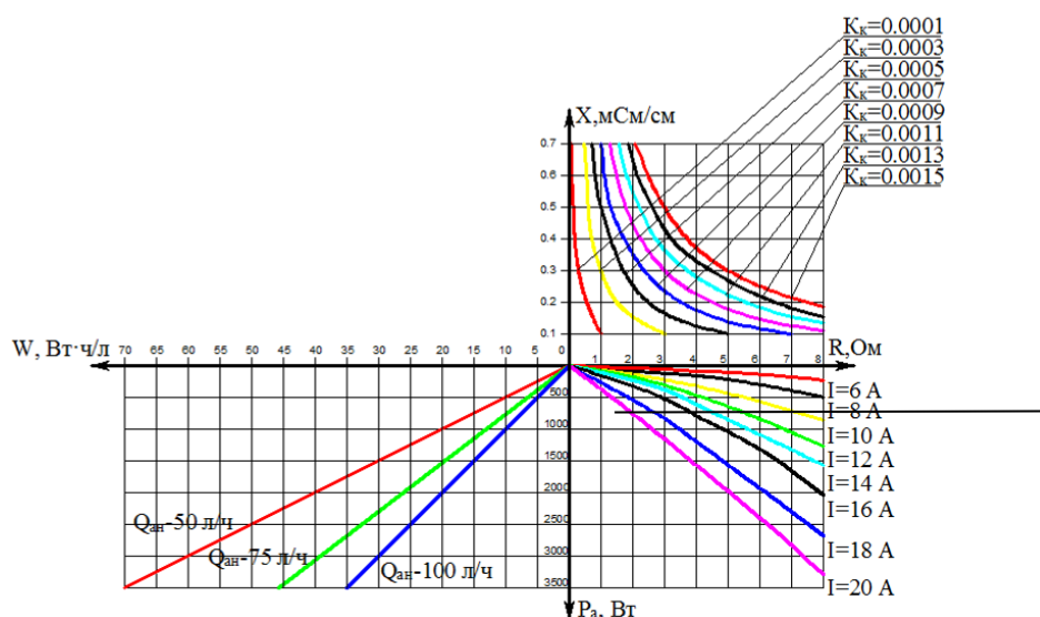
Рисунок 3.29 – Номограмма зависимости электропроводности, сопротивления и расхода электроэнергии при различной силе тока, конструктивном параметре и производительности
