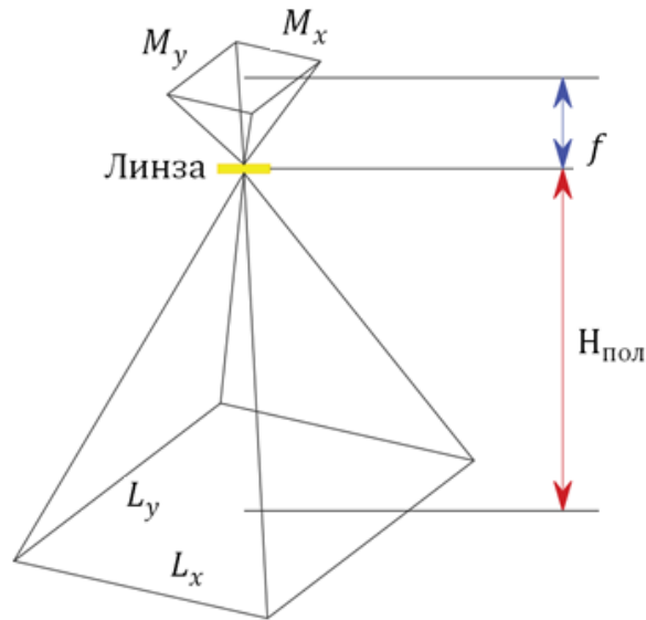
Рисунок 2.28 – Изображение связи ширины и длины матрицы на размер кадра
