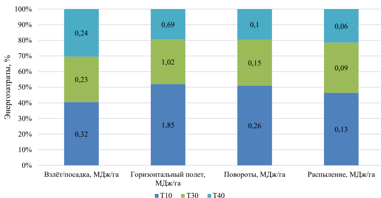
Рисунок 4.24 – Гистограмма энергопотребления БАС по элементам
