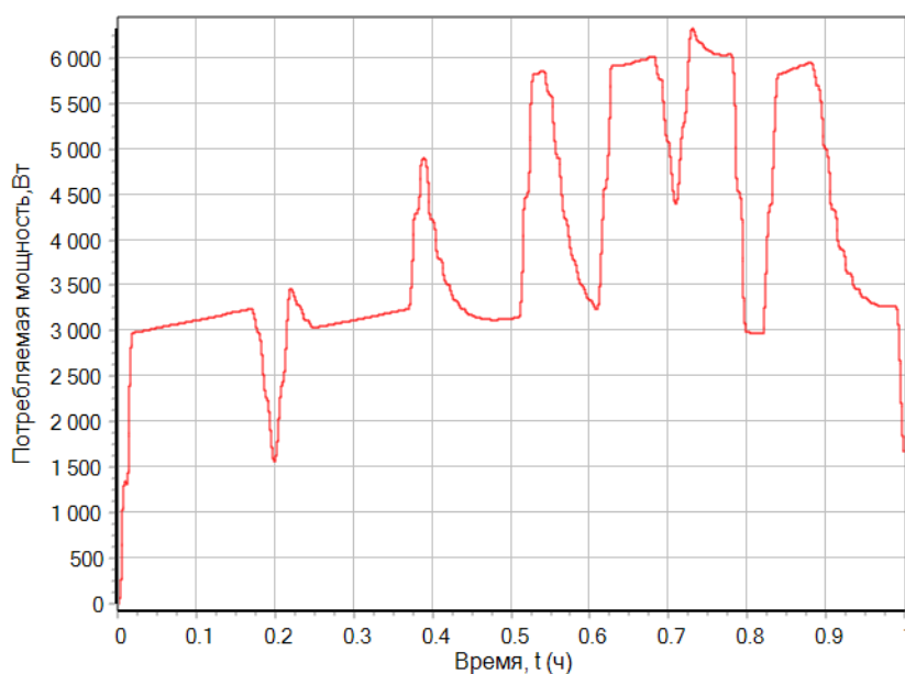
Рисунок 2.34 – График потребляемой мощности при поточном зарядке АКБ
