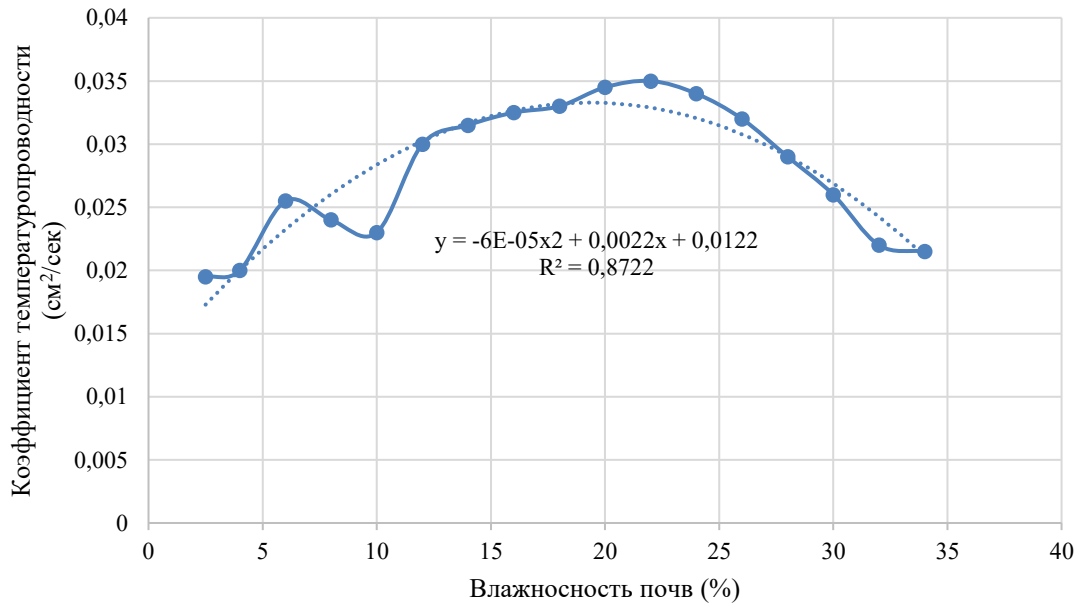
Рисунок 2.11 – График определения коэффициента температуропроводности почвы
