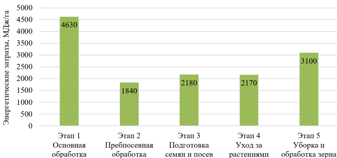
Рисунок 2.2 – Диаграмма энергозатрат по этапам возделывания пшеницы
