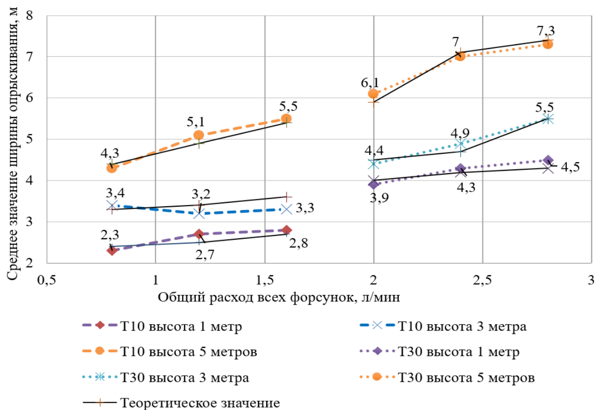
Рисунок 4.19 – График зависимости ширины обработки от высоты полета и расхода рабочего раствора
