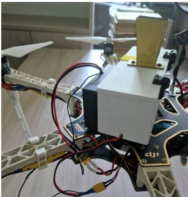
Рисунок 1.11 – Изображение пробоотборника воздуха
