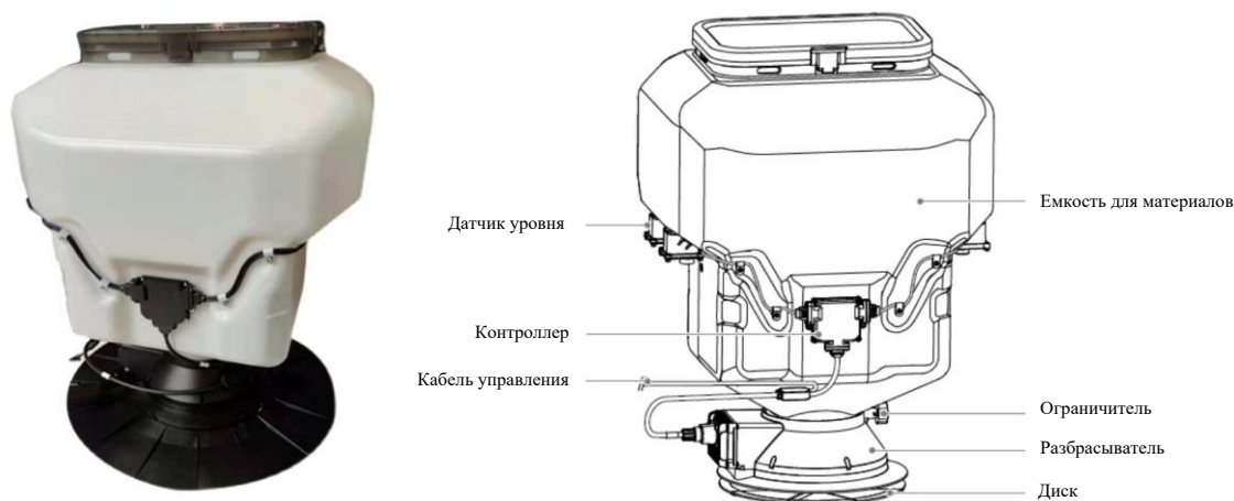
Рисунок 1.18 – Изображение внешнего вида системы разбрасывания
