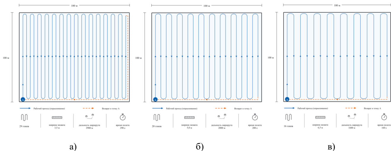
а) – DJI T10; б) – DJI T30; в) – DJI T40 Рисунок 4.23 – Изображение схем пролета при опрыскивании 1 га
