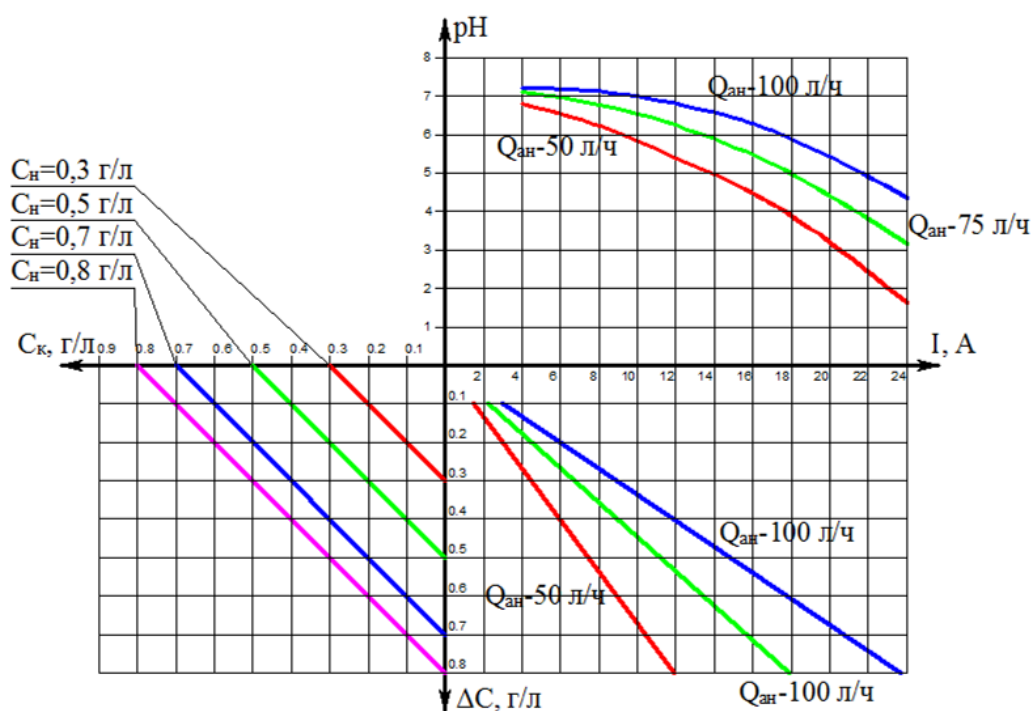
Рисунок 3.27 – Номограмма зависимости \text{pH} раствора от тока и конечной минерализации при различной производительности и начальной минерализации
