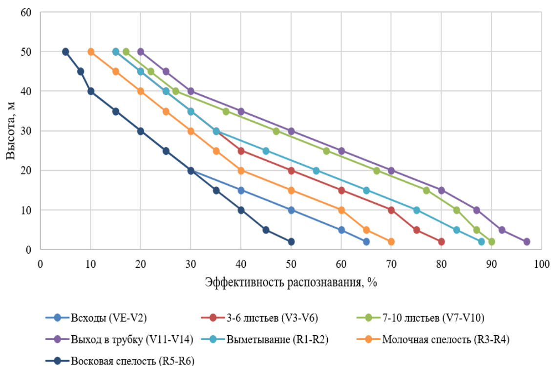
Рисунок 3.18 – График зависимости эффективности распознавания кукурузы в различных фазах
