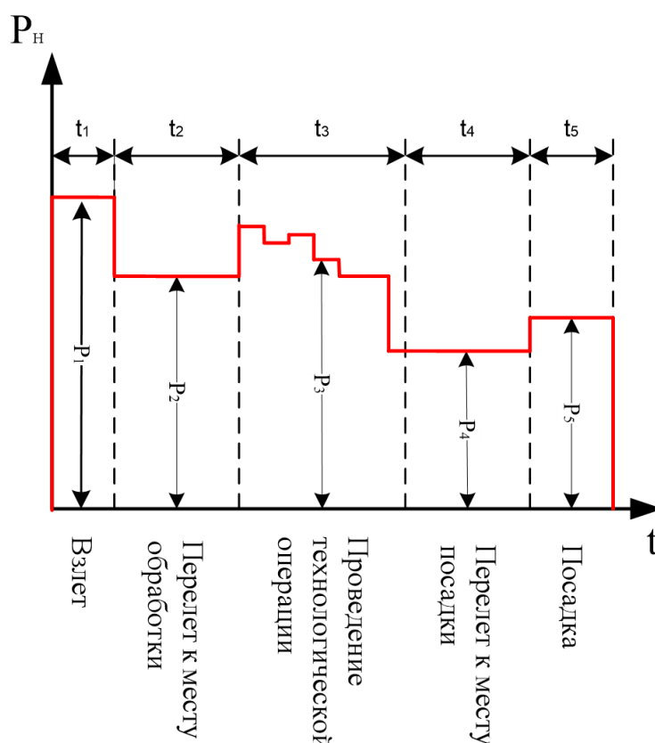
Рисунок 2.4 – Общий вид циклограммы нагрузок во время полета по галсам
