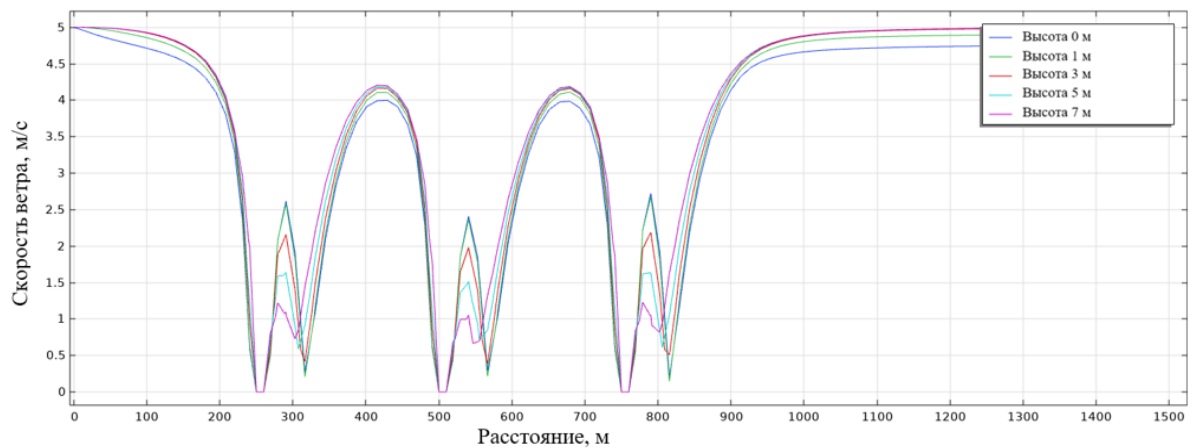
Рисунок 2.16 – График распределения скорости ветра на разных высотах при скорости набегающего потока 5 м/с
