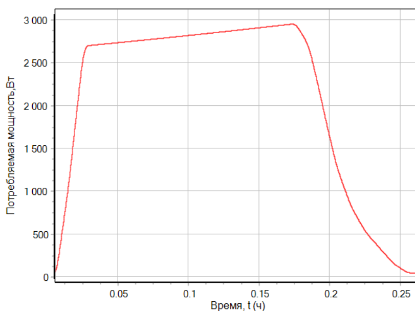
Рисунок 2.33 — График потребляемой мощности при зарядке одной АКБ БАС
