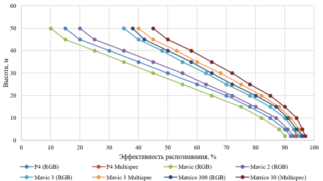
Рисунок 3.20 – График зависимости эффективности распознавания для различных БАС
